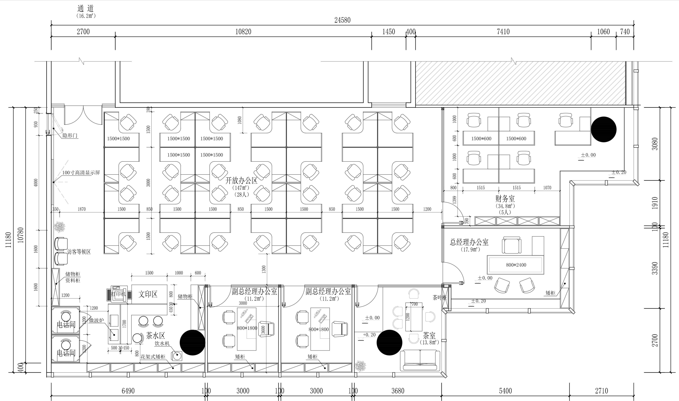
平面布置图 1:80
