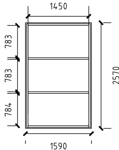
平面图
