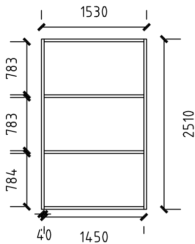
槽钢结构平面图
