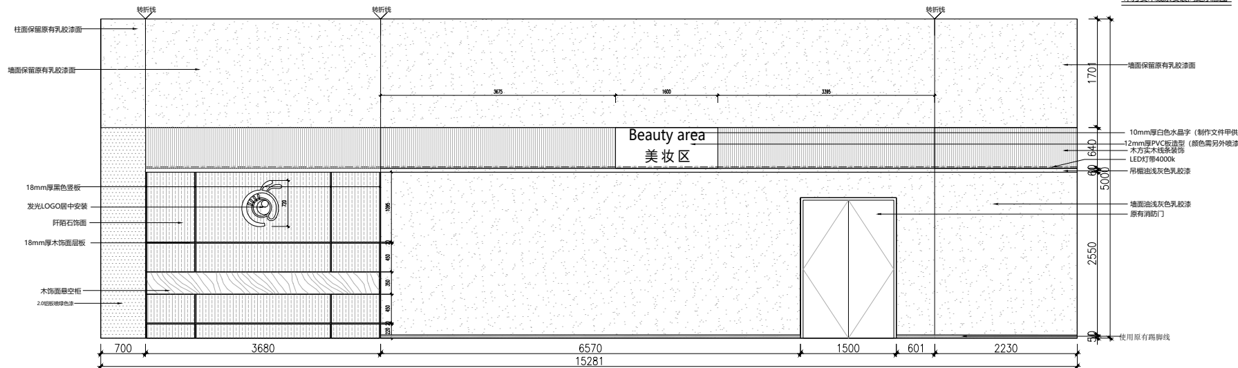
木方实木线条安装间距示意图
