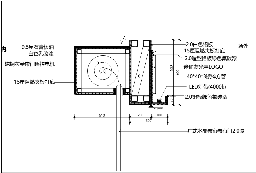
门楣节点图
