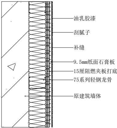
新建轻钢龙骨石膏板 隔墙刷漆工艺图
