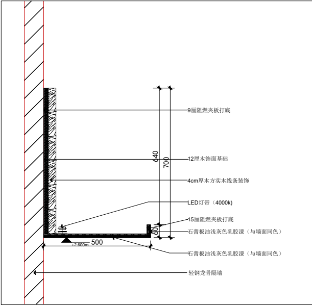
天花柜楣节点图
